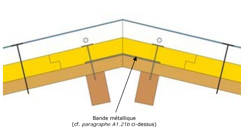
Figure 9 – Principe de jointolement du procédé Stisolétanch® Protect avec élément porteur bois - panneaux à base de bois, sur appui unique du faîtage ou arêtier
