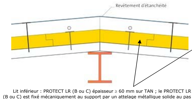
Figure 5 – Principe de jointoiement du procédé Stisolétanch® Protect avec élément porteur tôle d'acier nervurée, sur appui unique du faitage ou arêtier
