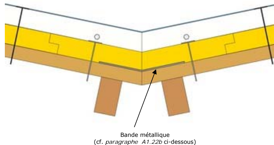
Figure 10 – Principe de jointolement du procédé Stisolétanch® Protect avec élément porteur bois - panneaux à base de bois, sur appui double de la noue en bois
