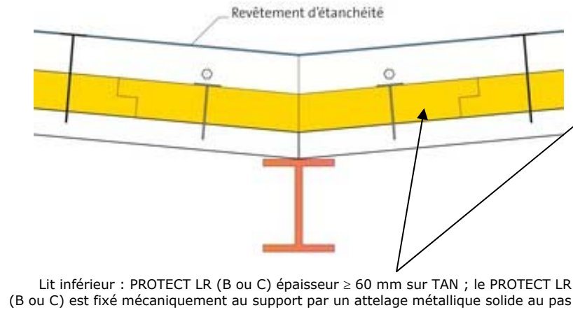
Figure 7 – Principe de jointoiment du procédé Stisolétanch® Protect avec élément porteur tôle d'acier nervurée, sur appui unique de noue traditionnelle
