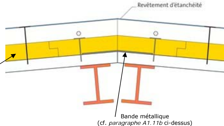
Figure 6 – Principe de jointoiement du procédé Stisolétanch® Protect avec élément porteur tôle d'acier nervurée, sur appui double du faitage ou arêtier
