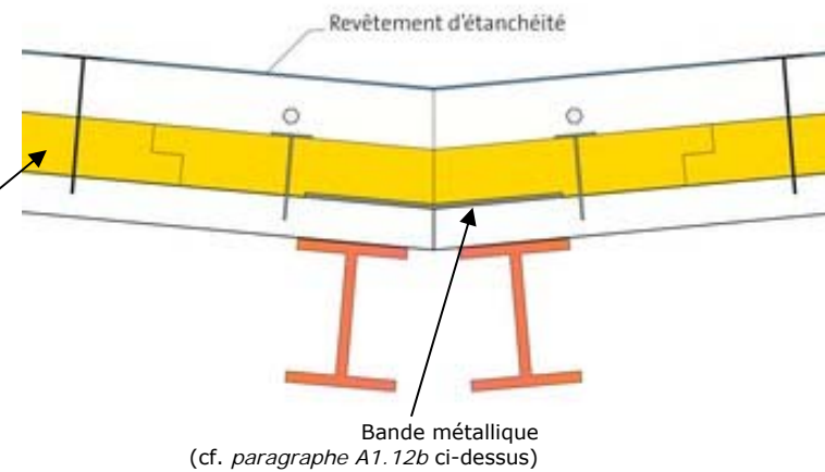
Figure 8 – Principe de jointoiment du procédé Stisolétanc® Protect avec élément porteur tôle d'acier nervurée, sur appui double de noue traditionnelle
